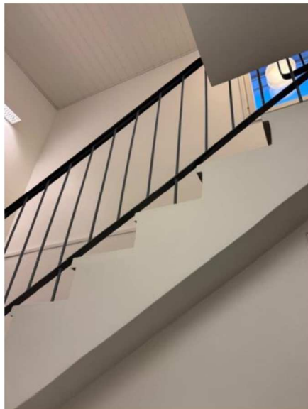
Kuva xx. Portaat ovat kapeat. Käsijohde on vain toisella puolella. Portaan etureuna on ulkovena.
