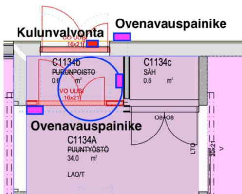
Kuva 1. Tuulikaappi ei ole suunnitelmassa esteetön. Pinkillä sähköisten ovenavauspainikkeiden (seinässä) paikat. Punaisella kulunvalvonnan paikka (viereisessä ovesta)
